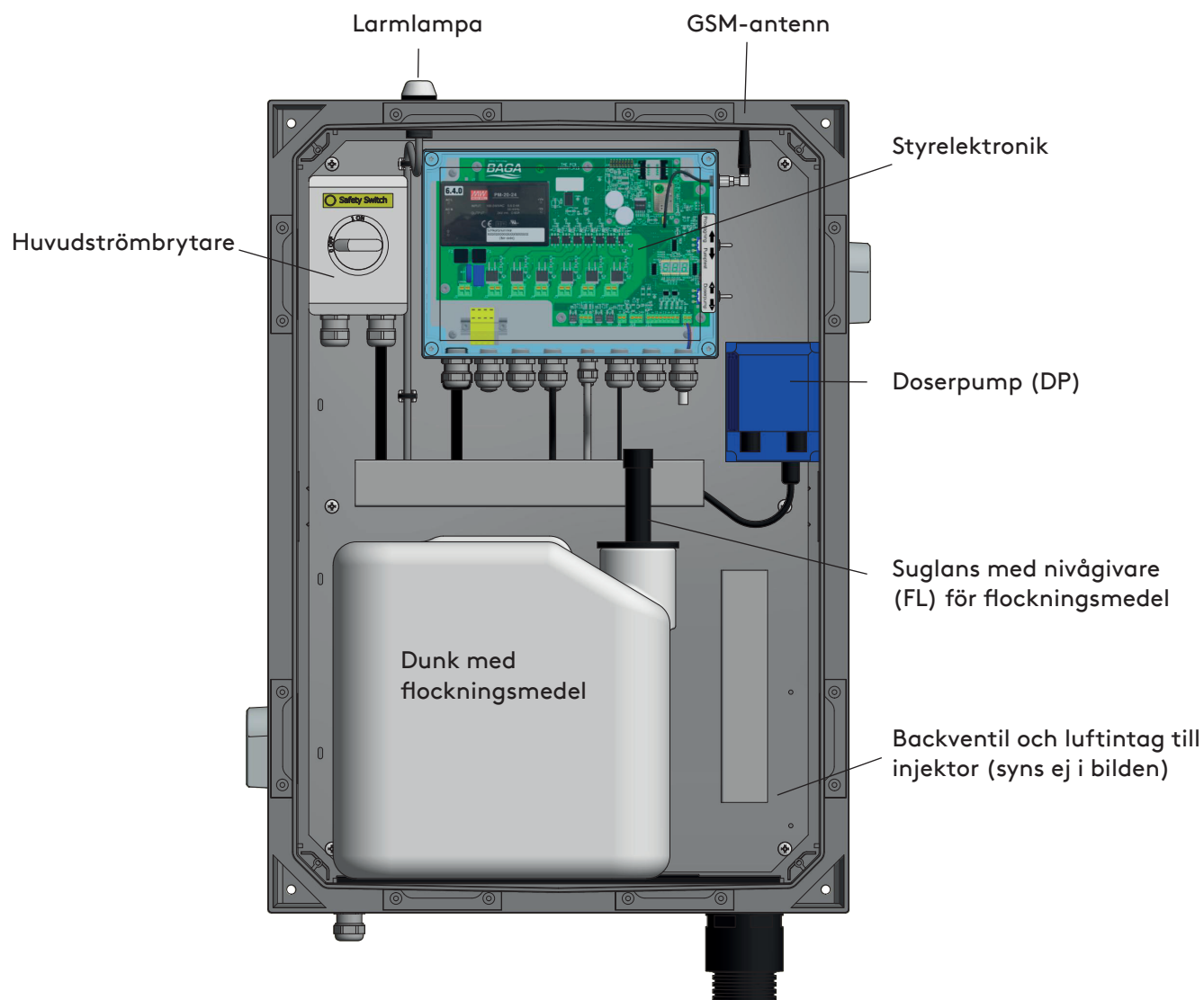
Figur 2. Översikt Automatikskåp
