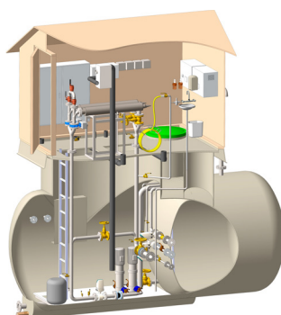
Vannbehandlingsanlegg med ventil/pumpe-kammer og vannbasseng opp til 100m 3 .
