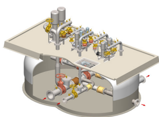
Trykkøkningsstasjon for vannforsyning
