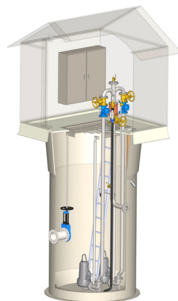
«Standard» pumpestasjon for avløp
